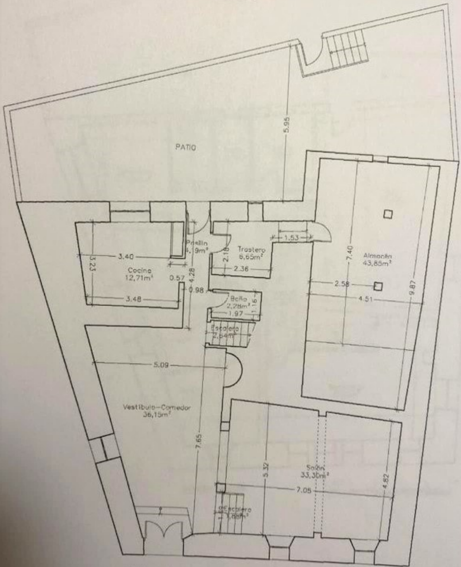
PLANTA BAJA
